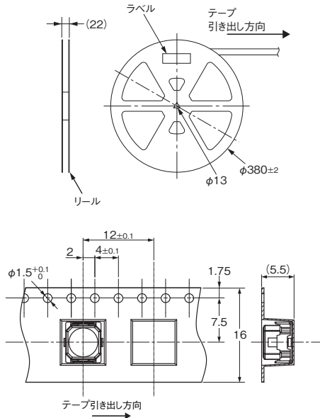
〈形B3ALの場合〉
