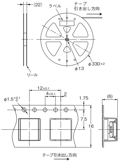
〈形B3FS-1092P/1095Pの場合〉
