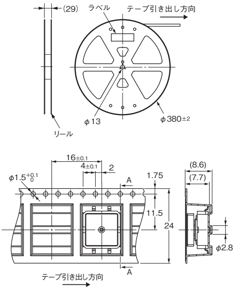
〈形B3FS-4092P-Bの場合〉
