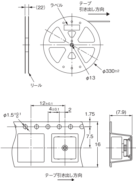
〈形B3FS-1092P-Aの場合〉
