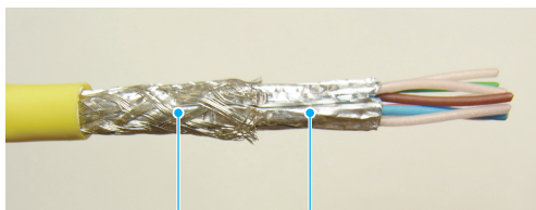
編組+アルミテープシールド
