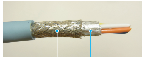
編組+アルミテープシールド
