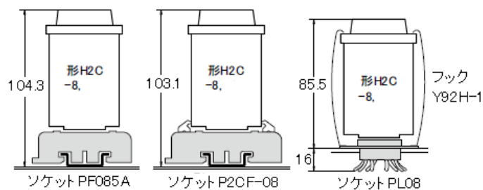
(表面取付時)
