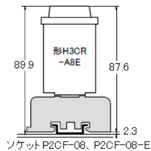
(表面取付時)
