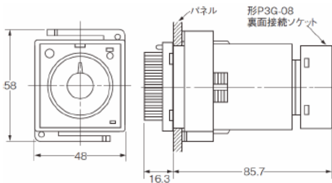
■外形寸法図 (埋込取付時)
