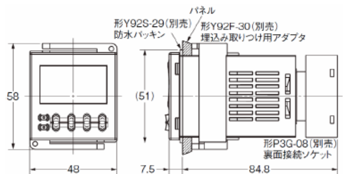
(表面取付時)
