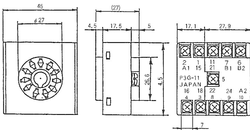
外形寸法図
