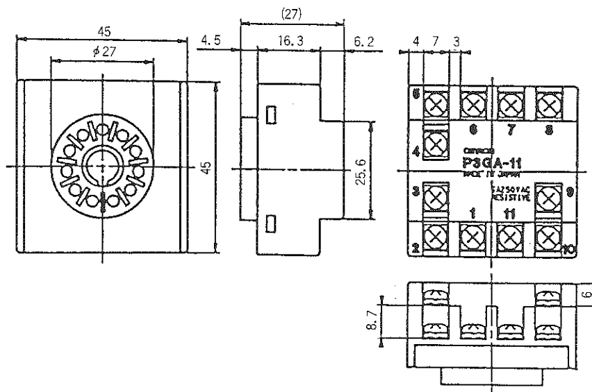
外形寸法図
