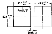
取り付け穴加工寸法
