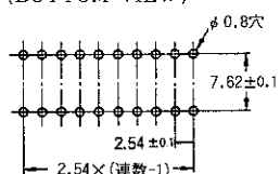
プリント基板加工寸法 (BOTTOM VIEW)
