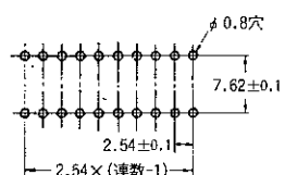
プリント基板加工図
