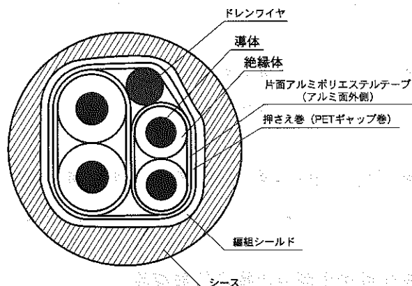
ケーブル断面
