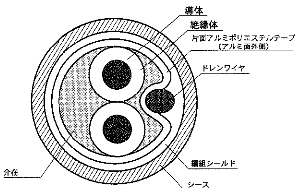
ケーブル断面
