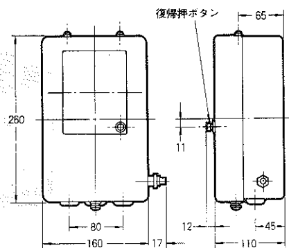
F4Aケース
