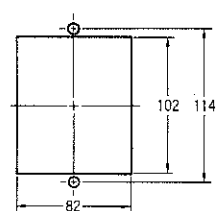
F2ケース
