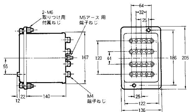
S8ケース
