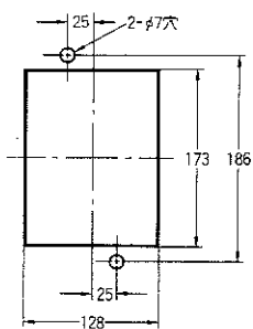
F4Aケース
