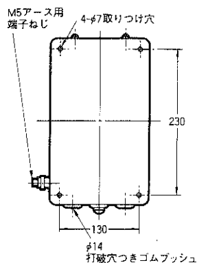
S8ケース
