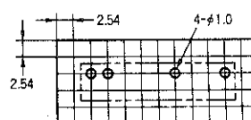
取付加工寸法 (BOTTOM VIEW)
