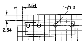
取付加工寸法 (BOTTOM VIEW)
