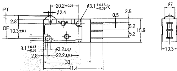
ピン押ボタン形(リード線タイプ)
