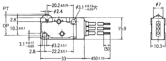
取付加工寸法
