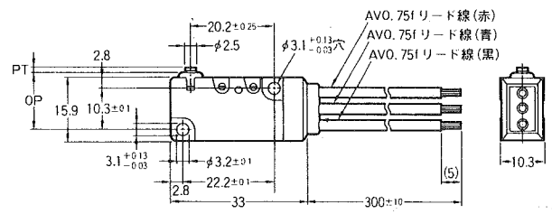
取付加工寸法
