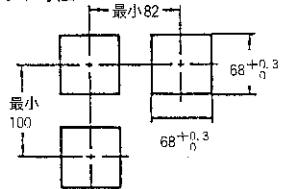
パネルカット寸法
