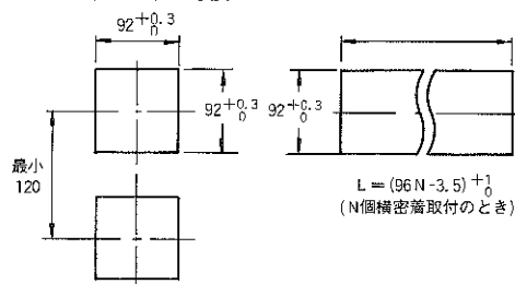
パネルカット寸法
