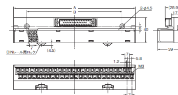
寸法表
