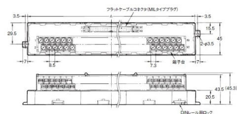
寸法表
