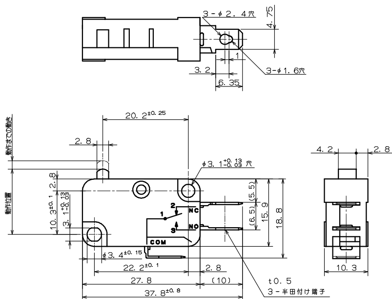
推奨代替商品 形V-10-1A4
