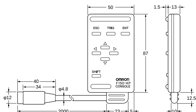
推奨代替商品 形F150-KP
