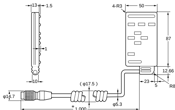
生産終了予定商品 形F300-KP
