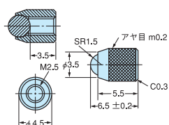
形D5SN-TB1/TB2/TB3
