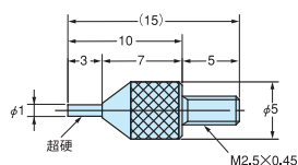
形D5SN-TN1
