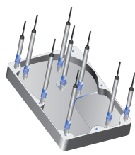
HDDシャーシの 反り測定
