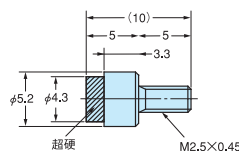
形D5SN-TF1
