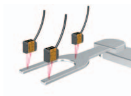
ロボットアームの 平坦度検査
