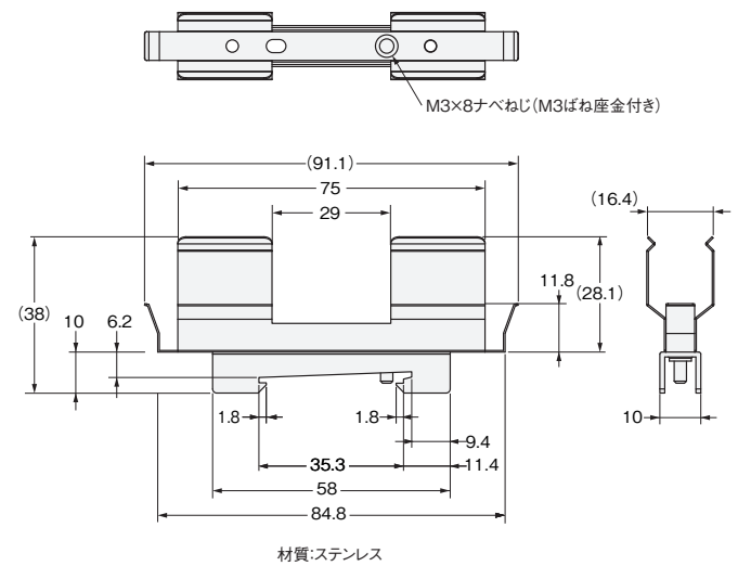
形ZX-XBT2 (DINレール取り付け用)
