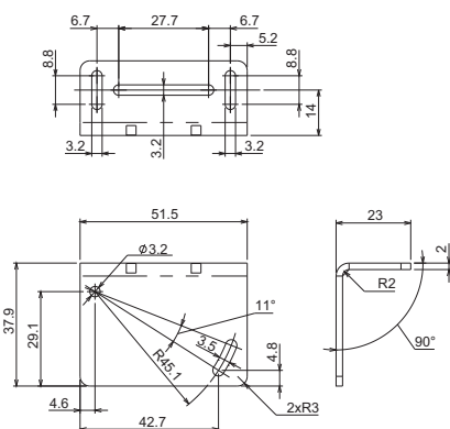
取付金具
