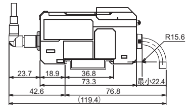
延長ケーブル(XS3W-M422/M424-□-□)接続時
