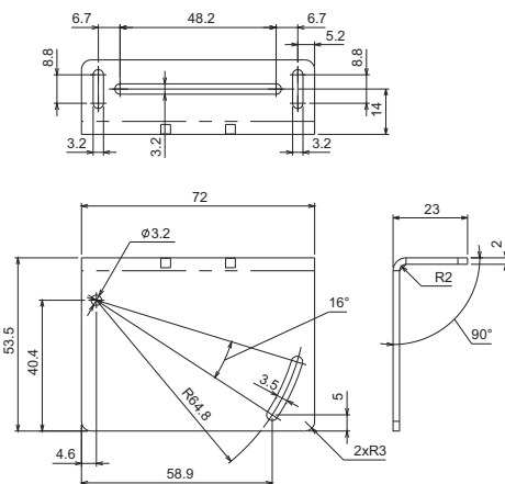
取付金具
