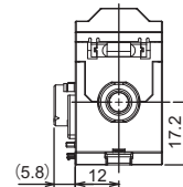
ユニット連結コネクタ位置
