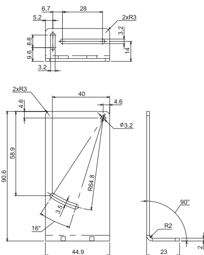
取付金具
