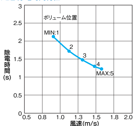
風速-除電時間特性
