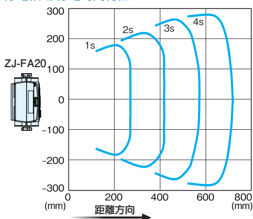
除電領域-除電時間特性
