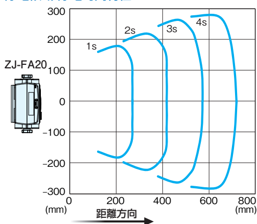
除電領域-除電時間特性
