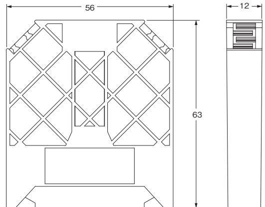
形XW5Z-EP12 (セパレートプレート)
