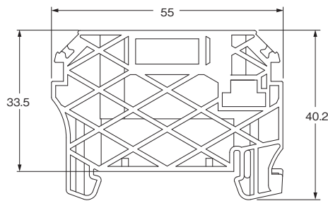
形XW5Z-EP6 (ストップ)
