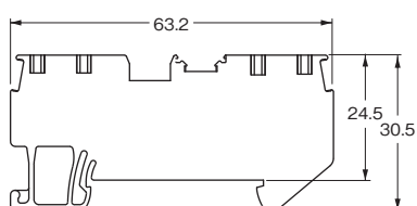
形XW5T-P2.5-1.1-1 (BL) / 形XW5G-P2.5-1.1-1
