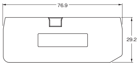
形XW5Z-EP6 (ストップ)
