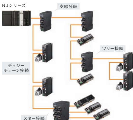
図1.配線例
