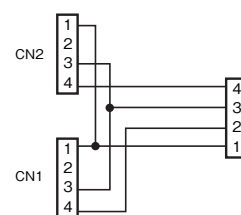
配線図
