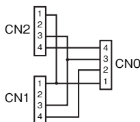
配線図
