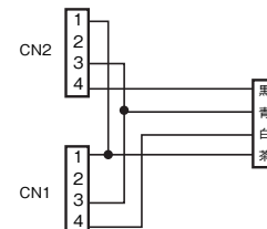
配線図
