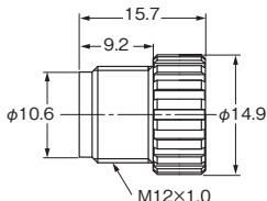
形XS2Z-22
