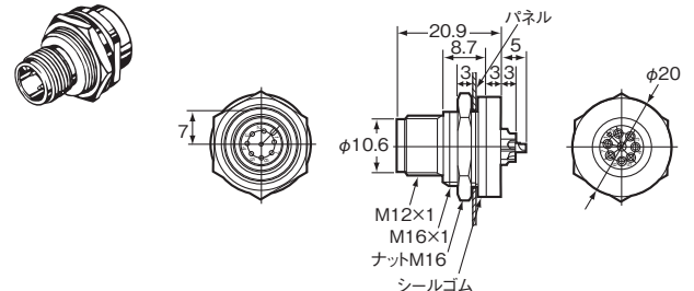
パネル取り付け用コネクタプラグ (M12) フロントロックタイプ 形XS2M-D824-4(溶ダーカップ端子)
