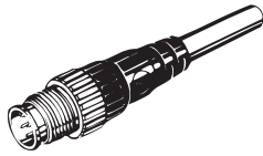
プラグ片側コネクタ (M12) 形XS2H
