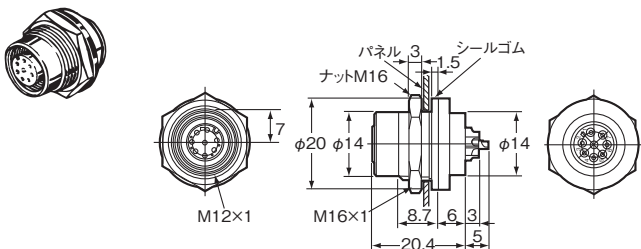
パネル取り付け用コネクタソケット (M12) フロントロックタイプ 形XS2P-D822-2(溶ダーカップ端子)
