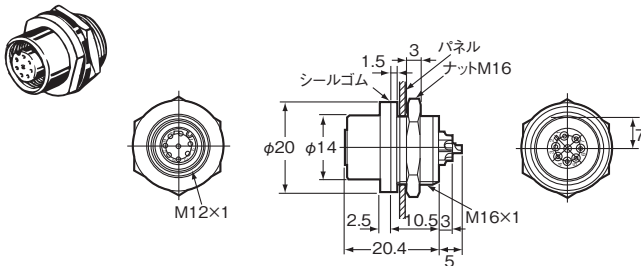
パネル取り付け用コネクタソケット (M12) フロントロックタイプ 形XS2P-D822-2(溶ダーカップ端子)
