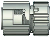
固定部バイonetロック機構拡大図
