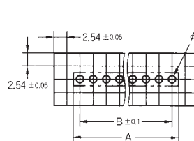
プリント基板加工寸法 (BOTTOM VIEW)
