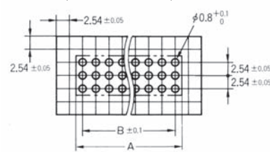
プリント基板加工寸法 (BOTTOM VIEW)
