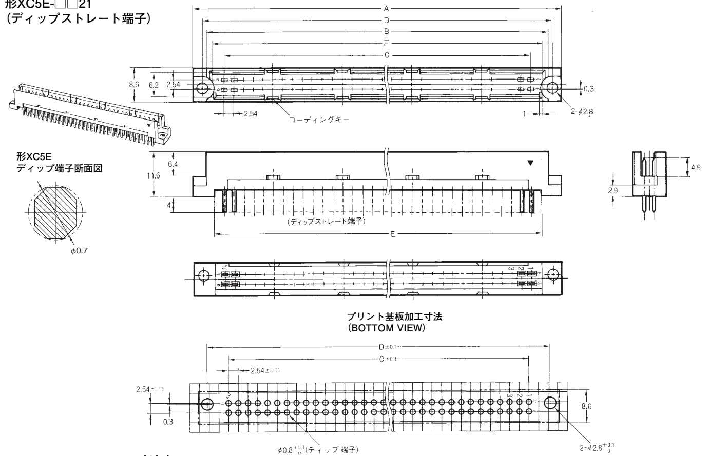
寸法表
