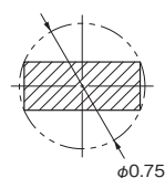
形XC5B ディップ端子断面図
