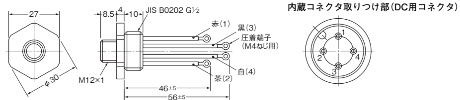
内蔵コネクタ取り付け部 (DC用コネクタ)
