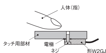
I字電極 (形W2GJ-F5)
