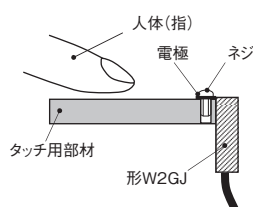
L字電極 (形W2GJ-L6)
