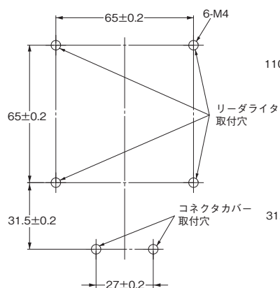
形V680S-HMD64-ETN、 形V680S-HMD64-EIP 取付穴加工寸法
