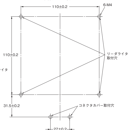
取付穴加工寸法
