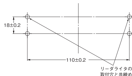
取付穴加工寸法
