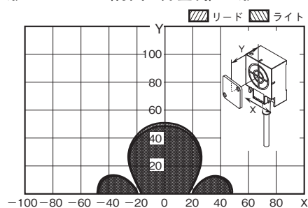
形V680-H01-V2(背面：非金属) & 形V680-D1KP66T(背面：非金属)
