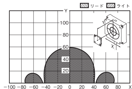
形V680-HS63(背面：金属) &amp; 形V680S-D2KF68(RFタグ横向き)
