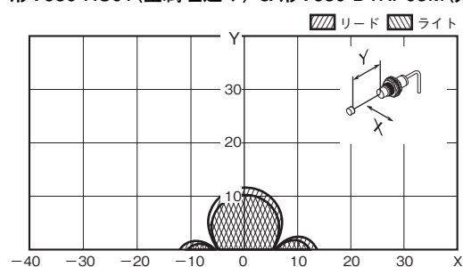
形V680-HS52(非金属埋込み) &amp; 形V680-D1KP53M(非金属埋込み)
