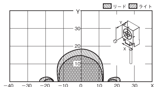
形V680-HS63(背面：非金属) & 形V680-D1KP66T(背面：非金属)
