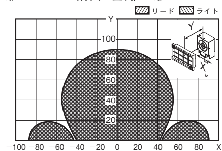
形V680-HS65(背面：金属) &amp; 形V680S-D2KF68(RFタグ横向き)
