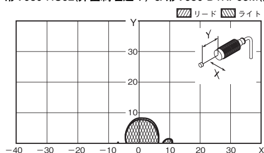
形V680-HS52(非金属埋込み) &amp; 形V680-D1KP53M(金属埋込み:鉄)
