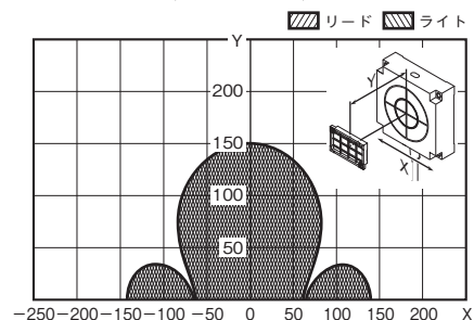
形V680-HS63(背面：金属) &amp; 形V680S-D2KF68M(RFタグ横向き)
