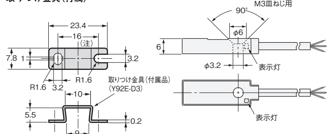
取り付け金具 (付属)
