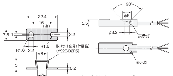
取り付け金具 (付属)
