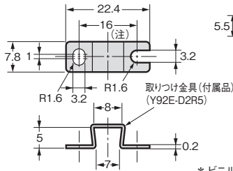
取り付け金具(付属)
