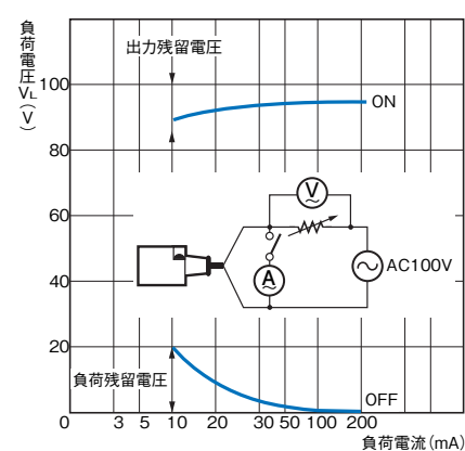
形TL-N□MY、AC100V時
