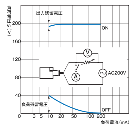
TL-N□MY AC200V時
