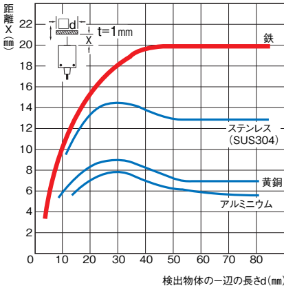
形TL-N20□
