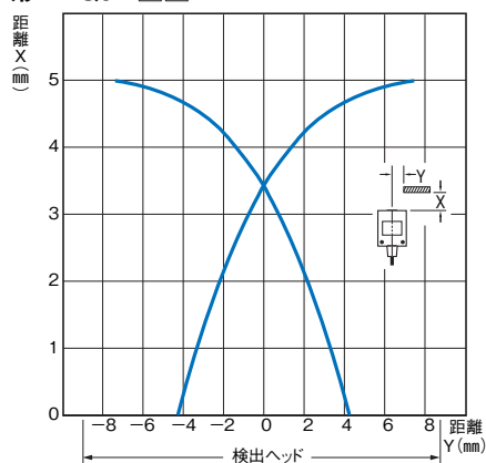
形TL-Q5M□□
