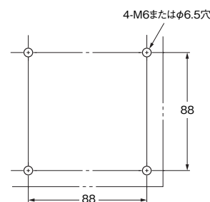
取り付け穴加工寸法
