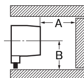
周囲金属の影響
