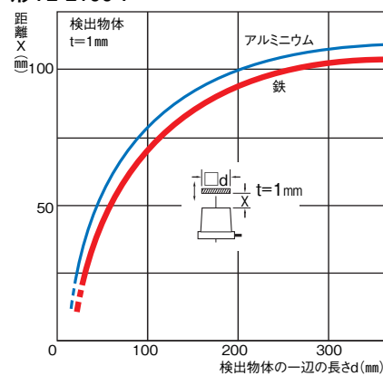
検出物体の大きさと材質による影響 形TL-L100-7
