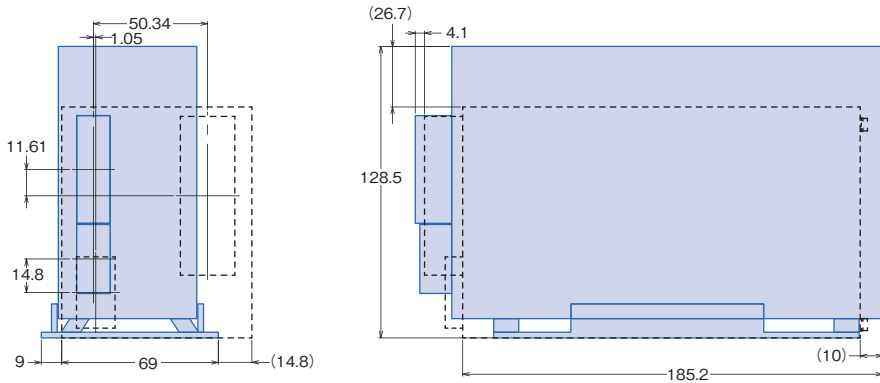
形S8VM-600□□
