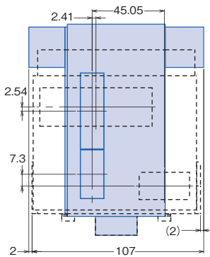
形S8VM-600□□
