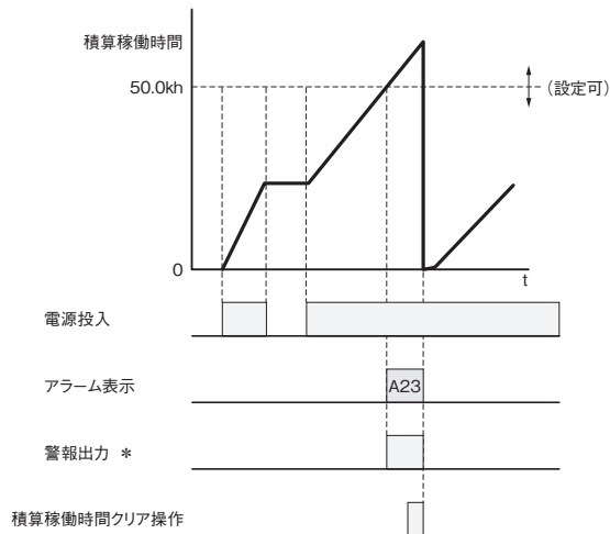
チャート(3) (動作イメージ)
