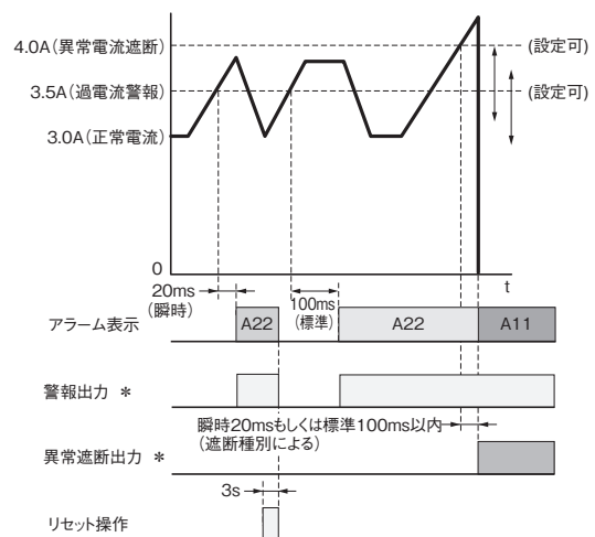
チャート(2) (動作イメージ)
