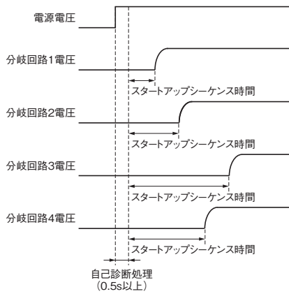
チャート(5) (動作イメージ)
