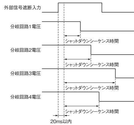
チャート(6) (動作イメージ)
