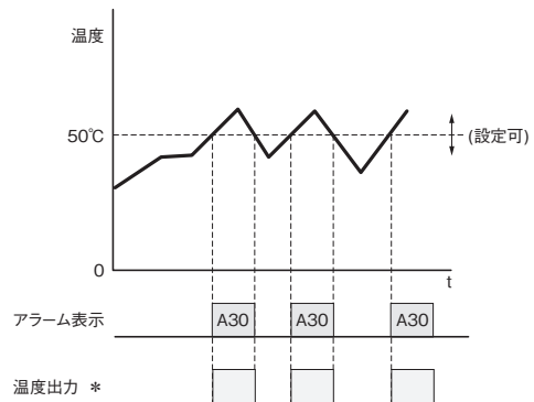
チャート(4) (動作イメージ)
