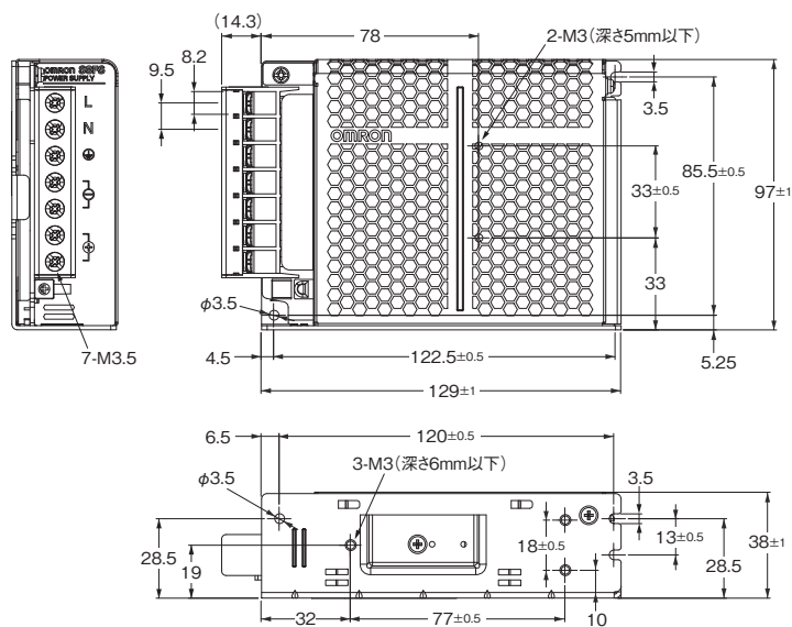
取り付け穴加工寸法
