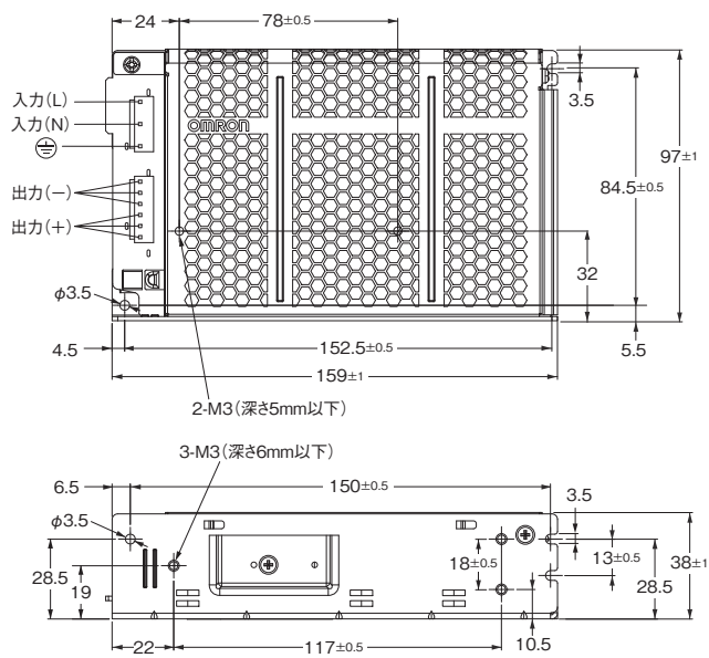
取り付け穴加工寸法
