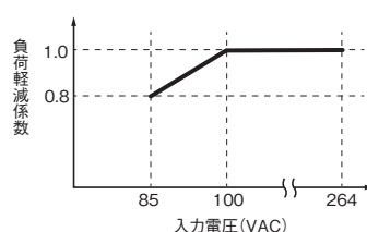
入力電圧に対する負荷軽減係数
