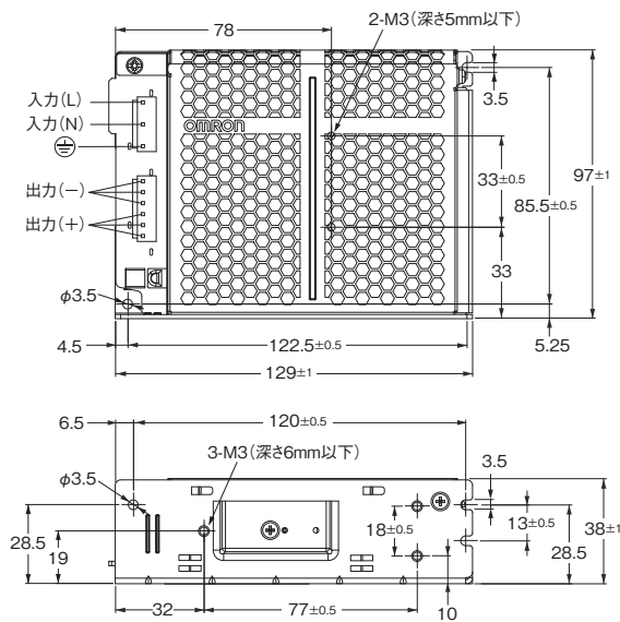
取り付け穴加工寸法
