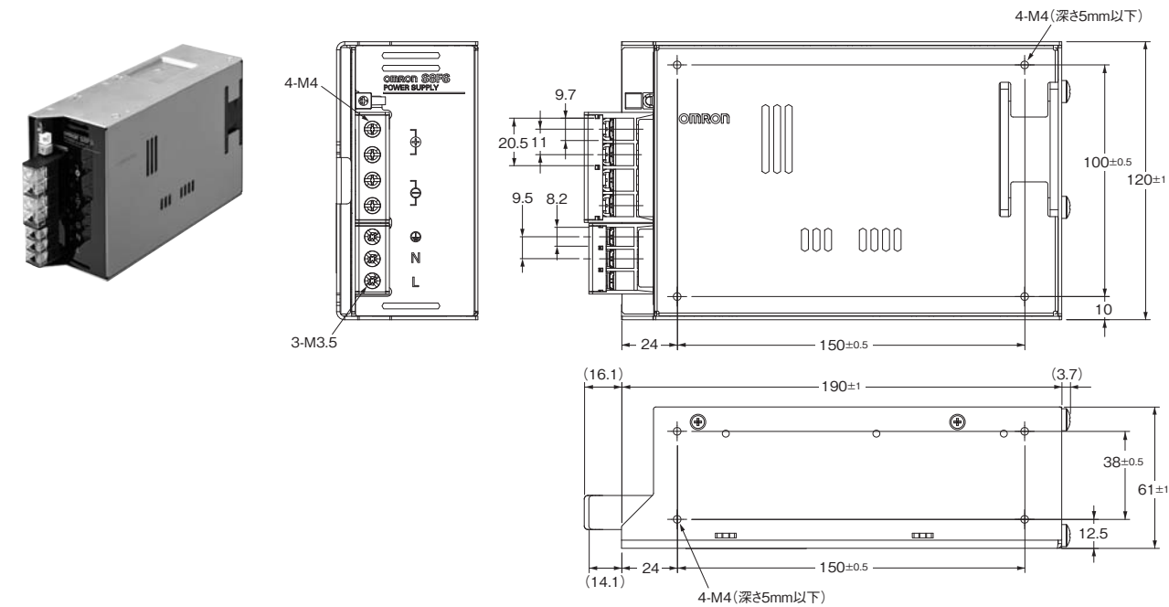
取り付け穴加工寸法
