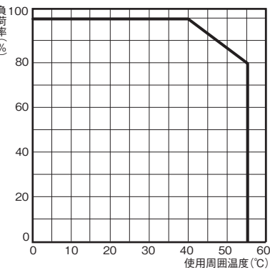
密着取り付け時(左右間隔0~15mm未満)
