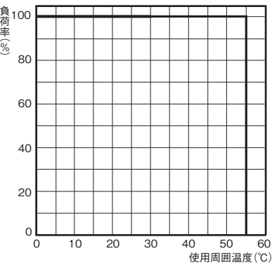
標準取り付け時(左右間隔15mm以上)
