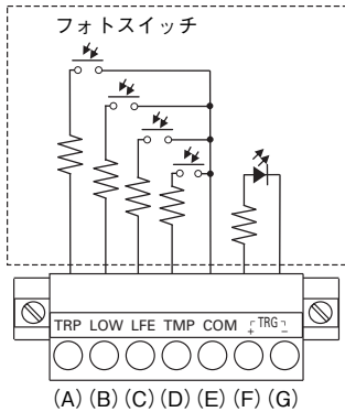
⑤入出力信号端子詳細 内部回路構成
