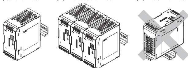
(A) 標準取り付け (B) 正面密着取り付け (C) 上向き取り付け
