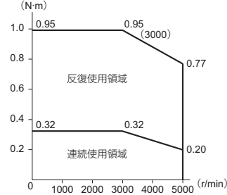
形R88M-G10030L
