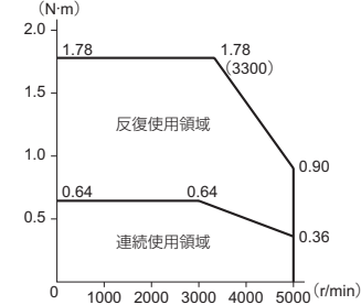
形R88M-G20030L
