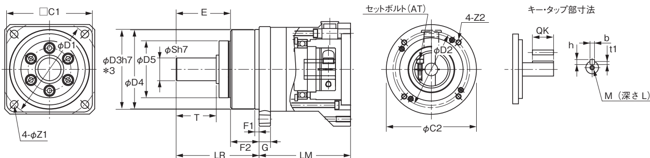
外形図2
