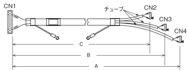
コネクタピン配置図 (コネクタかん合面より)
