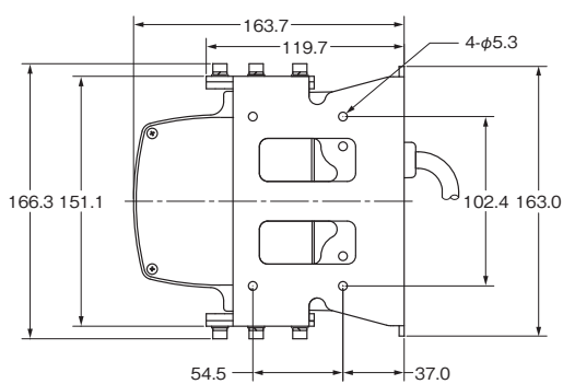
底面図
