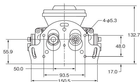
背面図 (背面取り付け用)
