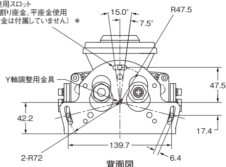
背面図 (Y軸角度調整用)
