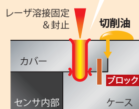
レーザー溶接イメージ
