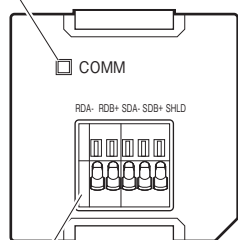
RS-422A/485端子台
