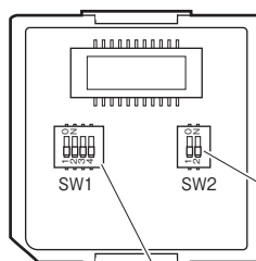
動作設定ディップスイッチ (SW1)
