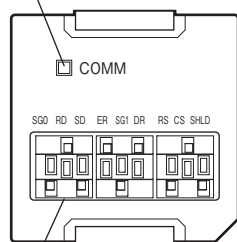
RS232C端子台
