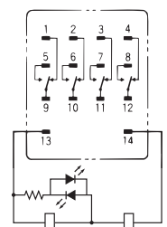
形MY4ZN-CBG (DC仕様)
