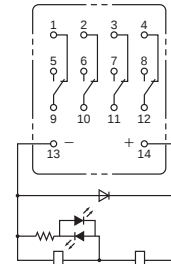
形MY4(Z) IN-D2(S) (DC仕様のみ)
