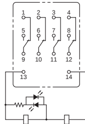
形MY4(Z) IN(S) (DC仕様)
