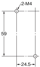
取り付け穴加工寸法
