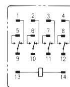
形MY4Z-CBG (AC/DC仕様)
