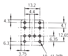
プリント基板加工寸法 (BOTTOM VIEW)
